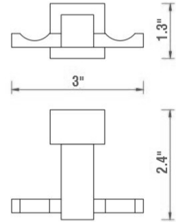
SBA-1582 | ROBE HOOK
